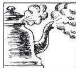
Газообразная – пар
