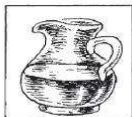
Жидкая
