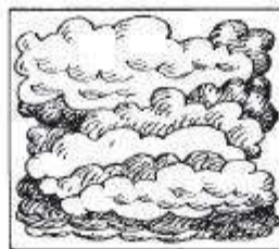
Облака
